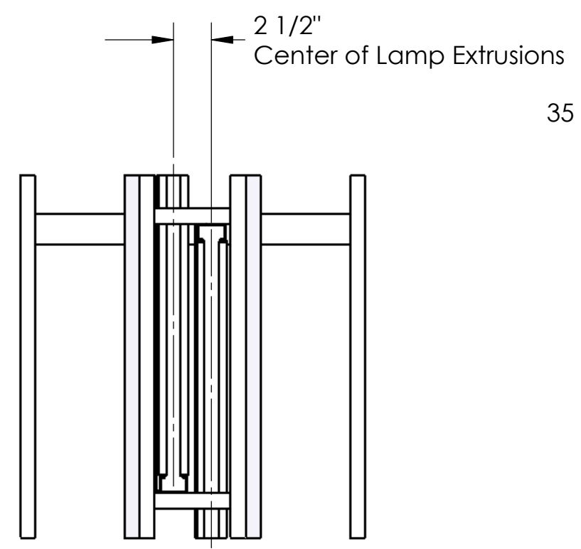
SECTION J-J SCALE 1 : 9
